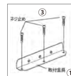
step 1 基本取付位置に合わせ取付金具をビスビス3本で固定します。
