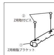
step 1 基本位置に合わせZ用樹脂ブラケットをZ用取付ビス2本で固定します。
